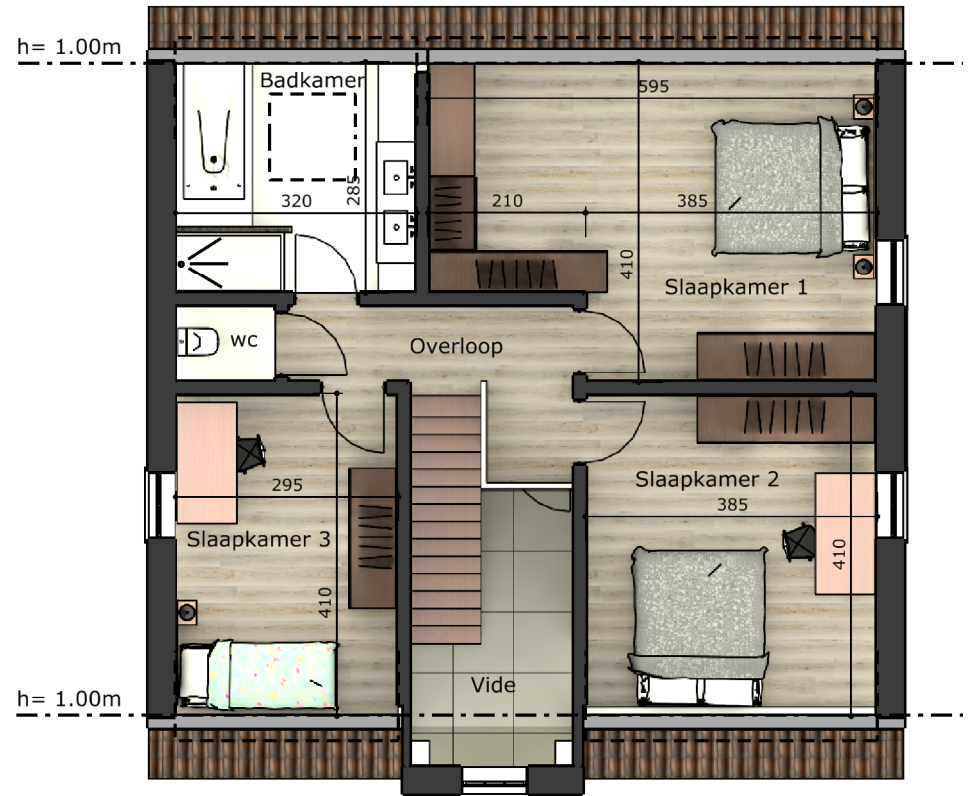
VERDIEPING Opp. verdieping 74 m 2 (min. hoogte 1.00m)
