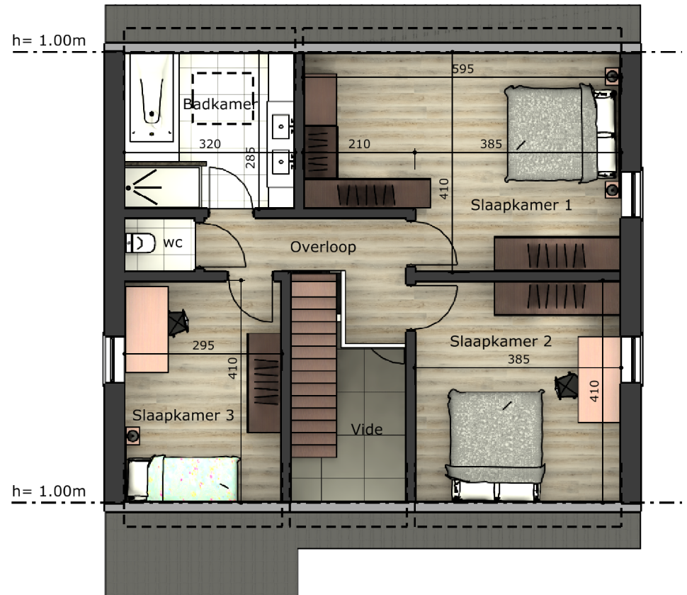
VERDIEPING Opp. verdieping 74 m 2 (min. hoogte 1.00m)
