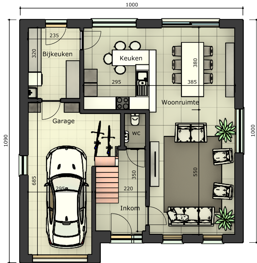
GRONDPLAN Opp. gelijkvloer 103 m 2
