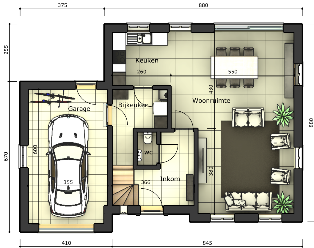
GRONDPLAN Opp. gelijkvloer 101,50m 2
