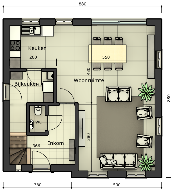
GRONDPLAN Opp. gelijkvloer 76m 2
