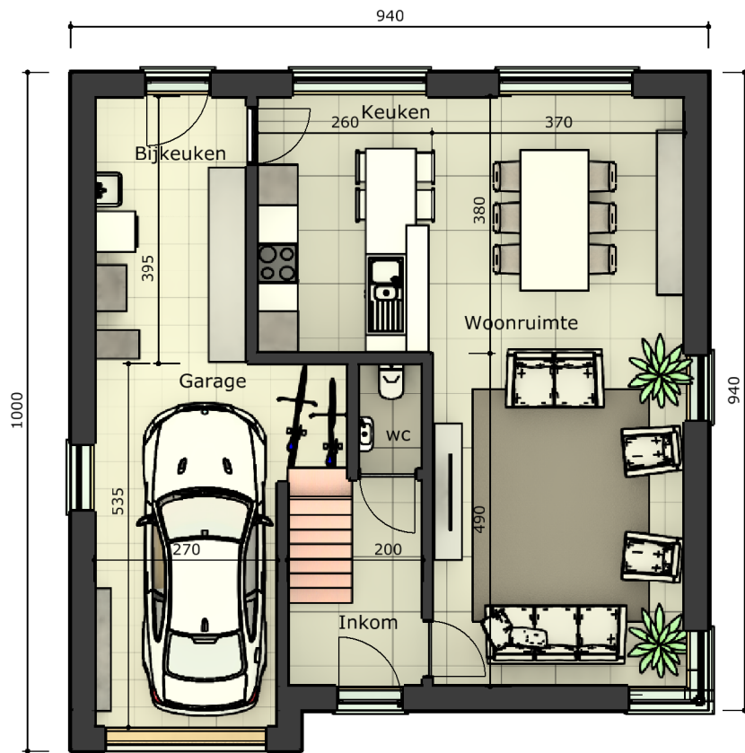
GRONDPLAN Opp. gelijkvloer 90.40 m 2
